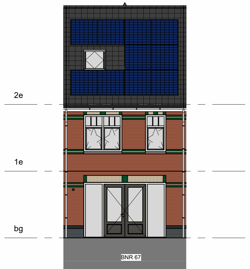
Achtergevel
