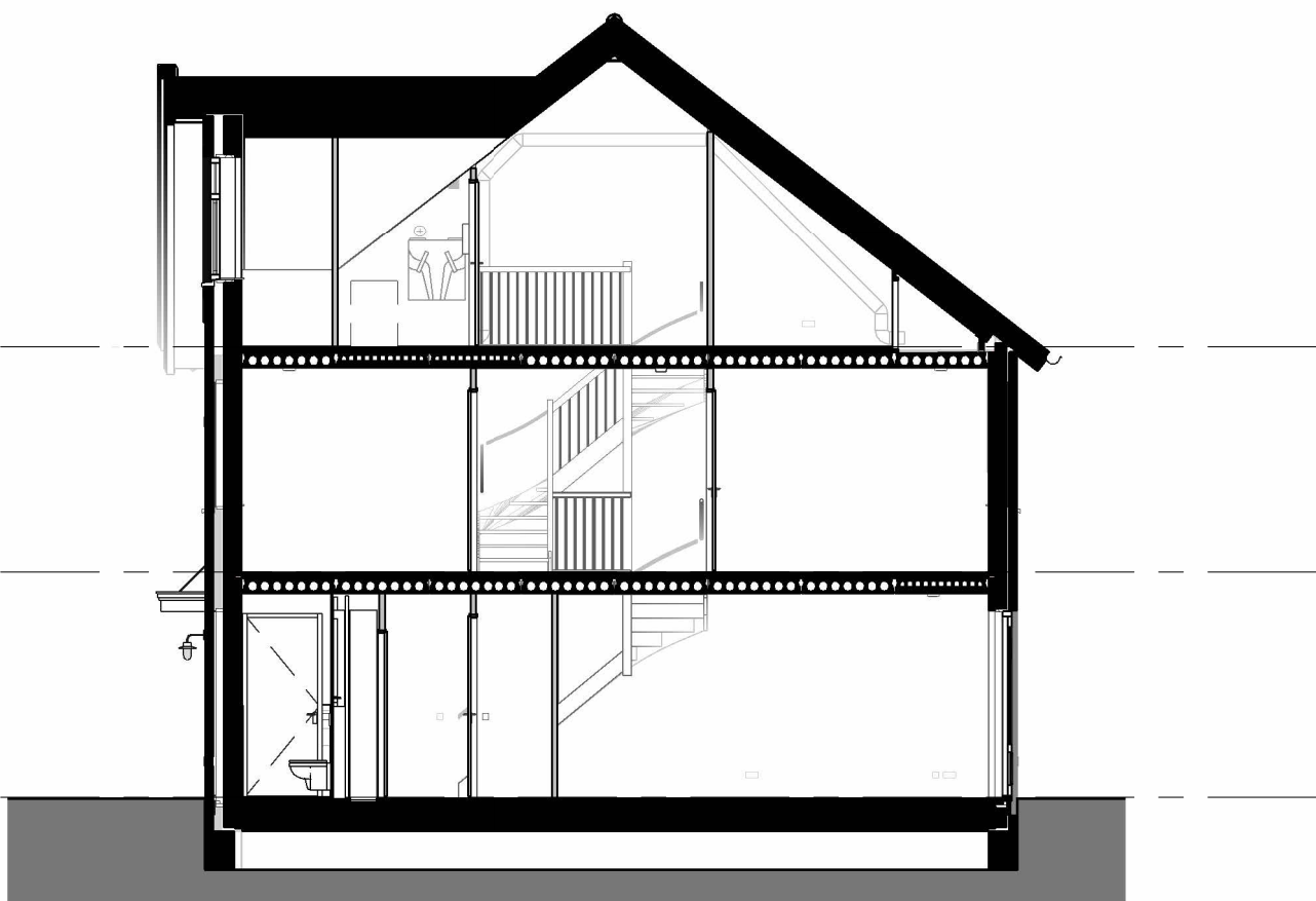
Doorsnede
