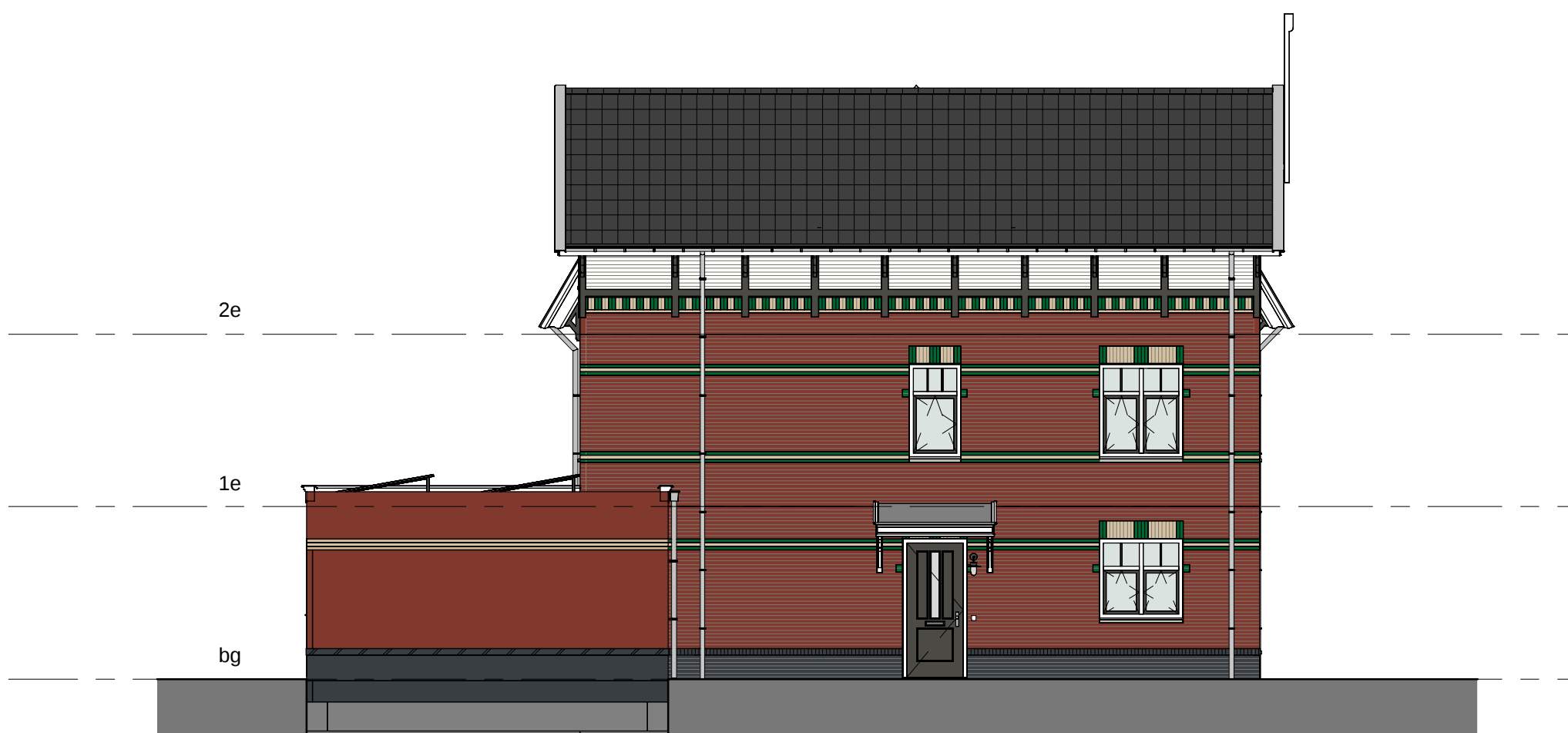
Linkergevel
