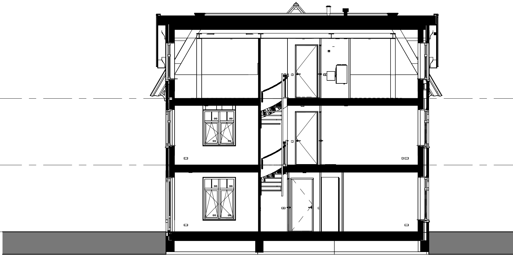
Doorsnede
