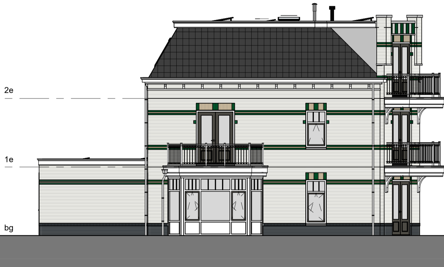
Linkergevel
