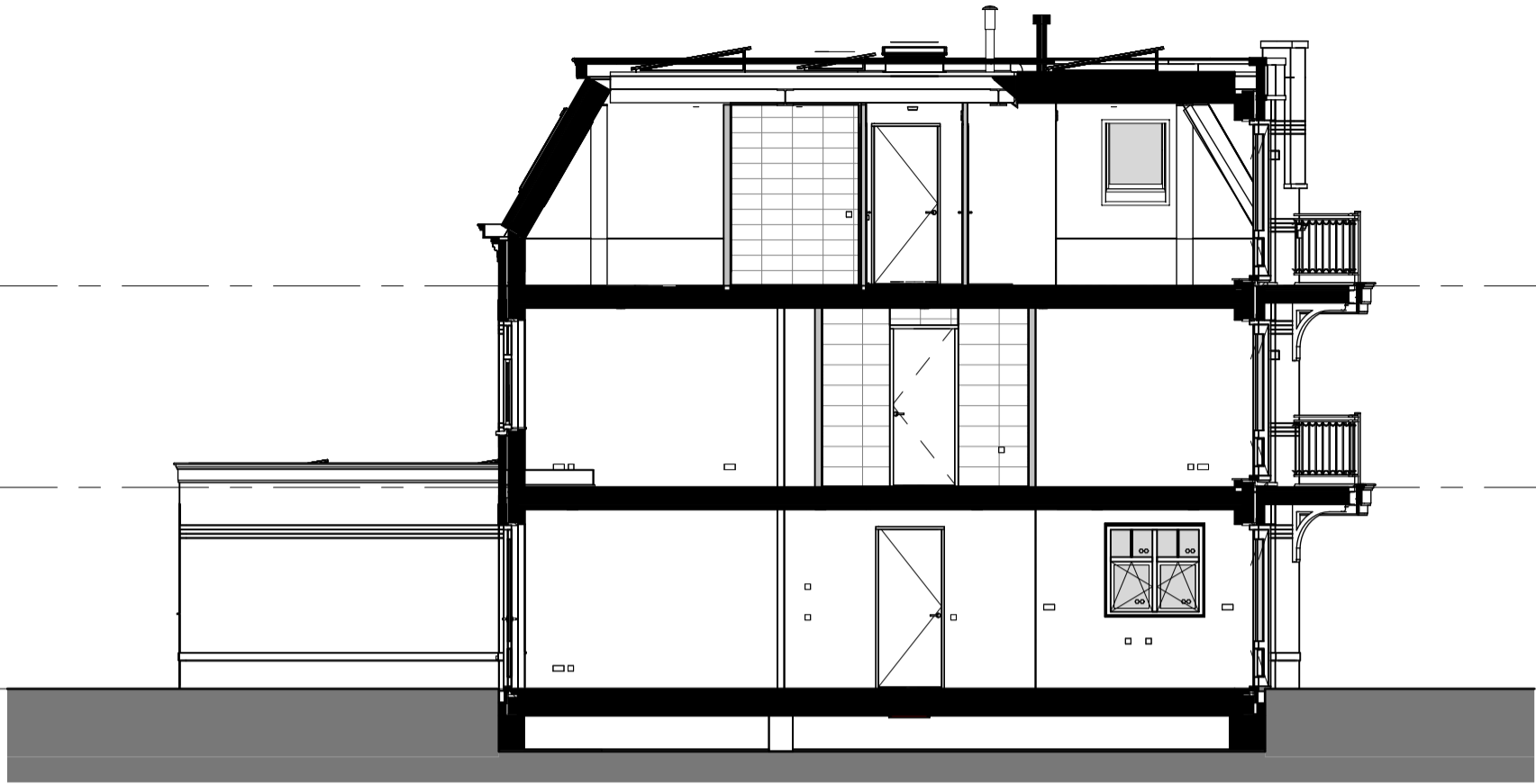
Doorsnede
