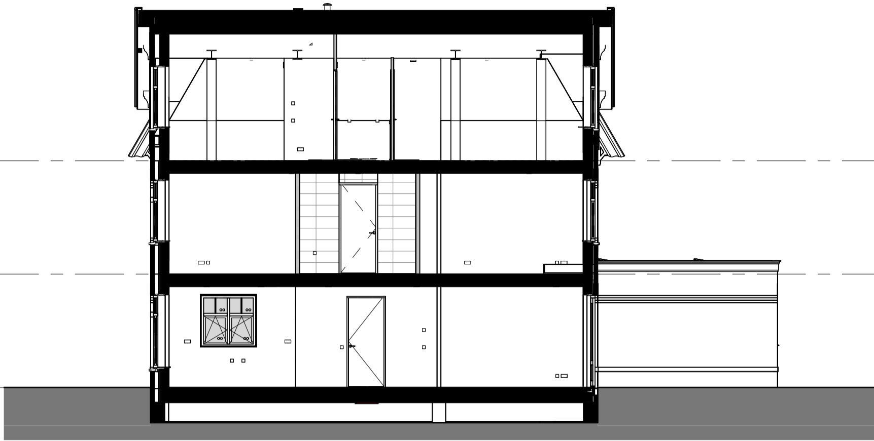
Doorsnede
