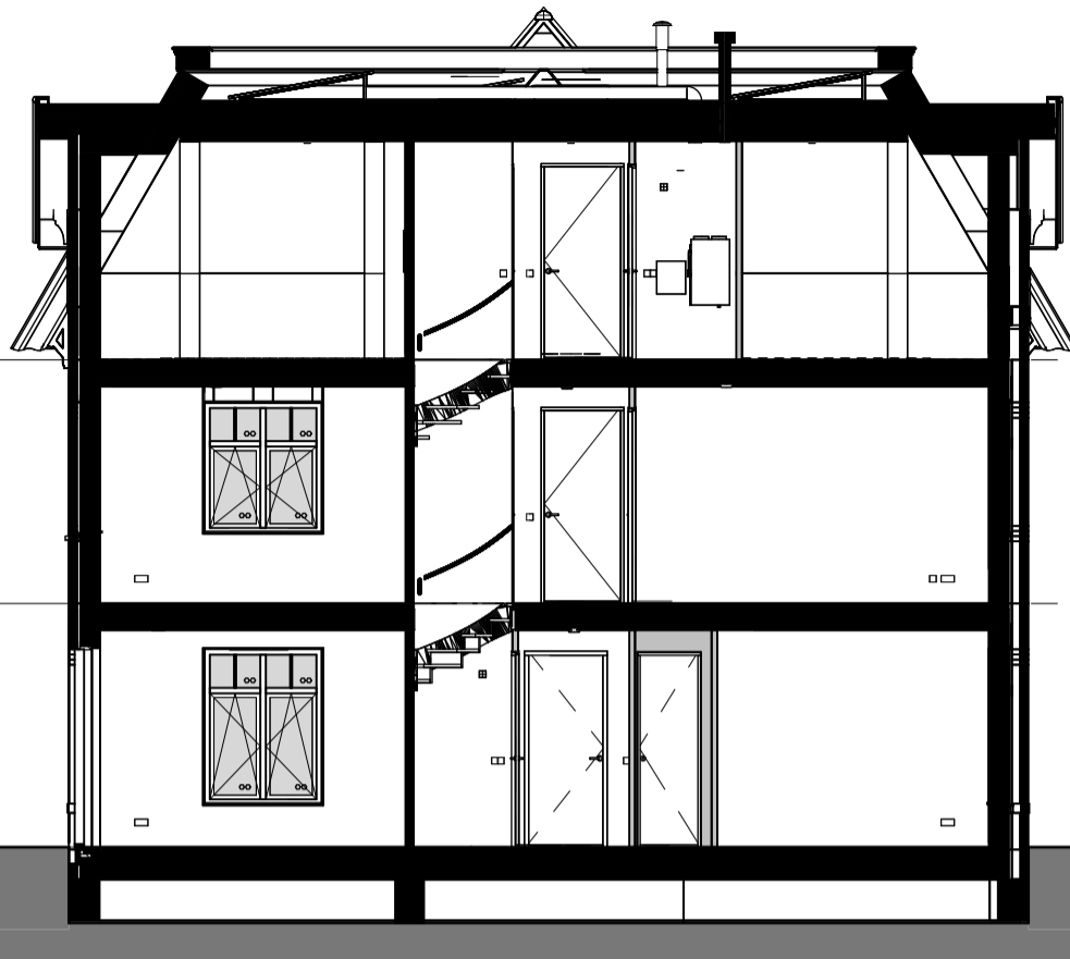
Doorsnede
