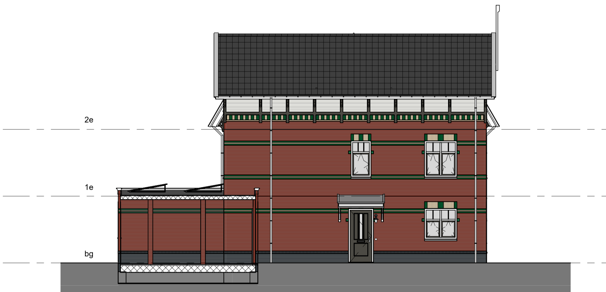
Linkergevel
